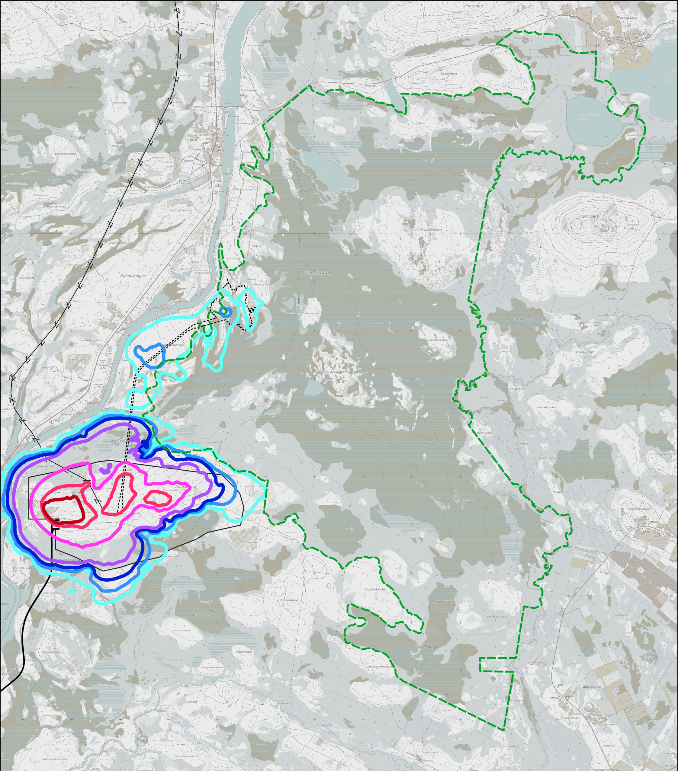
Pohjaveden alenema (m), 24 (heinäkuu) vuosi kaivostoiminnan aloittamisesta
