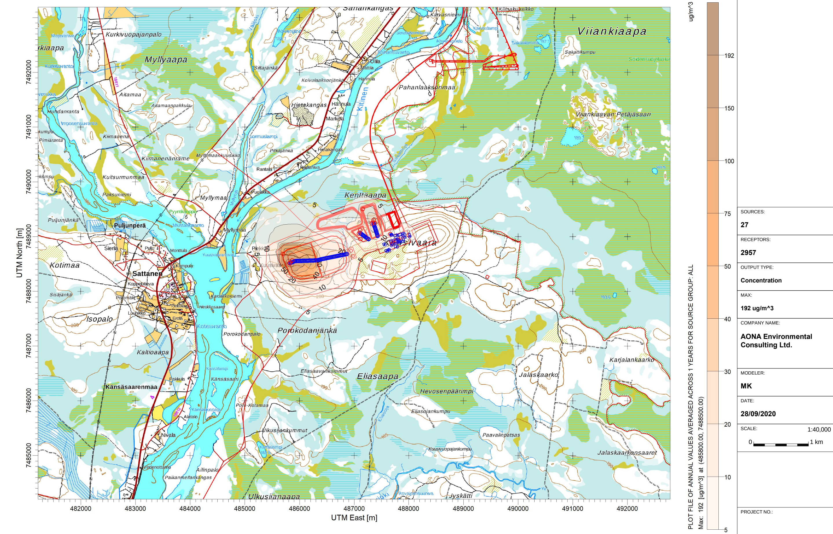
PROJEKTIN NIMI: Kuva 3: Sakatin kaivoshanke. Suunnitellun Sakatin kaivoshankevaihtoehtojen pölypäästöjen leviämismallinnus. Vaihtoehto VE3a - PM10 pitoisuuksien vuosikeskiarvo (µg/m3) - Vuosiraja-arvo hengitettäville hiukkasille = 40 µg/m3 (2017 Met data)
