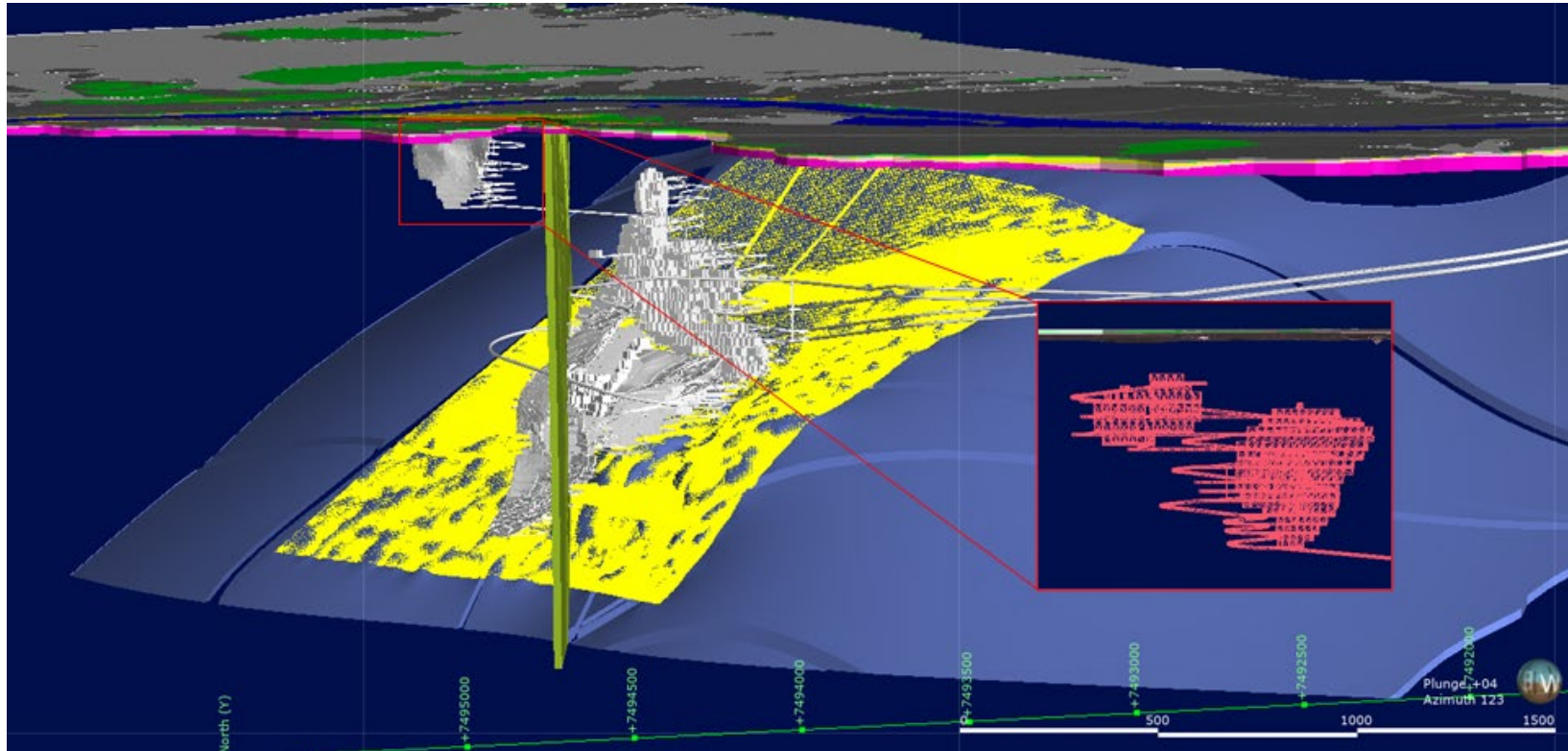
Kuva 6-21 Leapfrog-malli, jossa pohjasiirros suunnitellun kaivoksen jalkapuolet (footwall)
