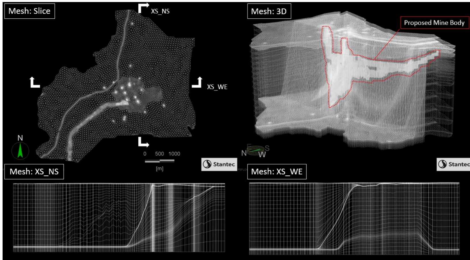
Kuva 6-6 Poikkileikkausnäköymä superhilaverkosta (vasen yläkulma) ja siirrosten sekä pohjan työntösiirroksen vertikaalisesta diskretoinnista FEFLOW-mallissa
