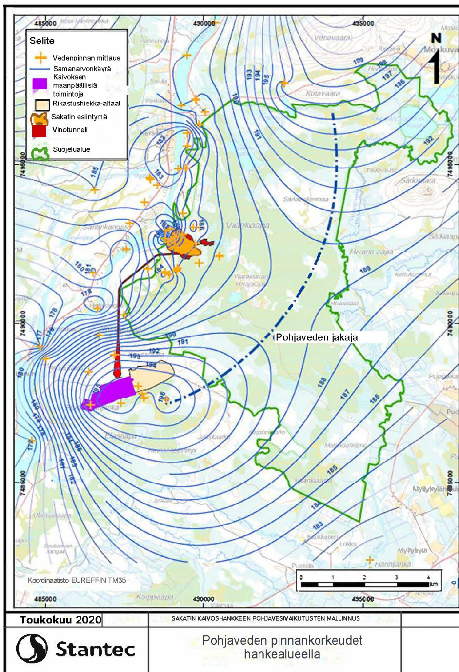
Kuva 2-9 Pohjavedenpinnan samanarvokäyrät jäätikkö- ja jokisyntyisissä sedimenteissä.
