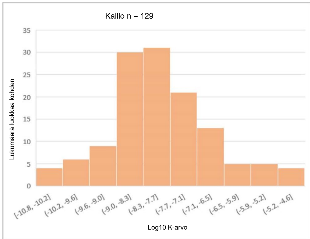
Kuva 2-13 Vedenjohtavuuskertoimen arvon vaihtelu terveessä, muuttumattomassa kallioperässä (SRK 2018, 2019)
