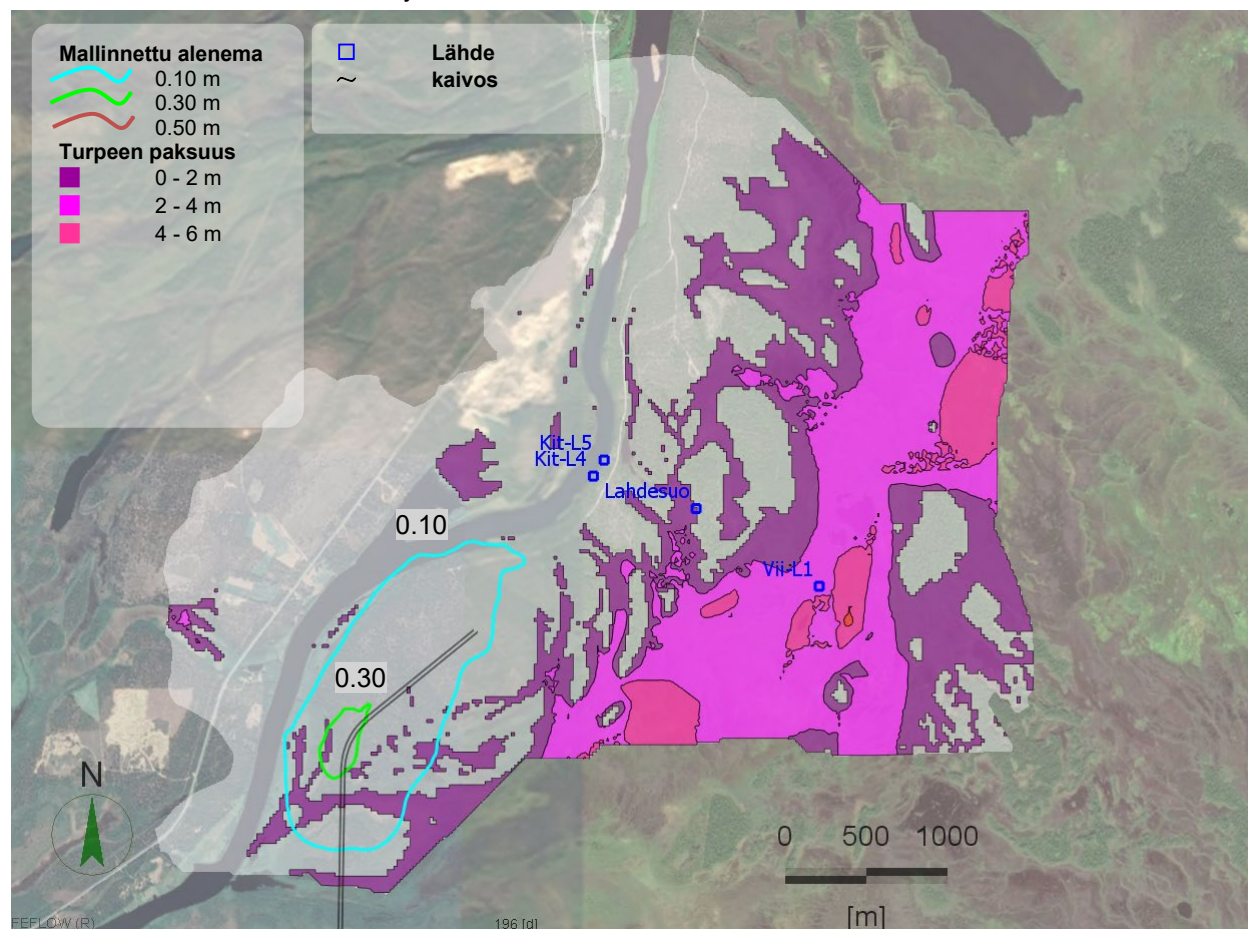
Kuva 8-1 Kaivos peruslievennystoimenpitein: Pohjaveden pinnan alennema mallin kerroksessa 1 (glasiaaliset ja fluviaaliset pintakerrokset ja turve) kaivostoiminnan vaiheessa Y-1.
