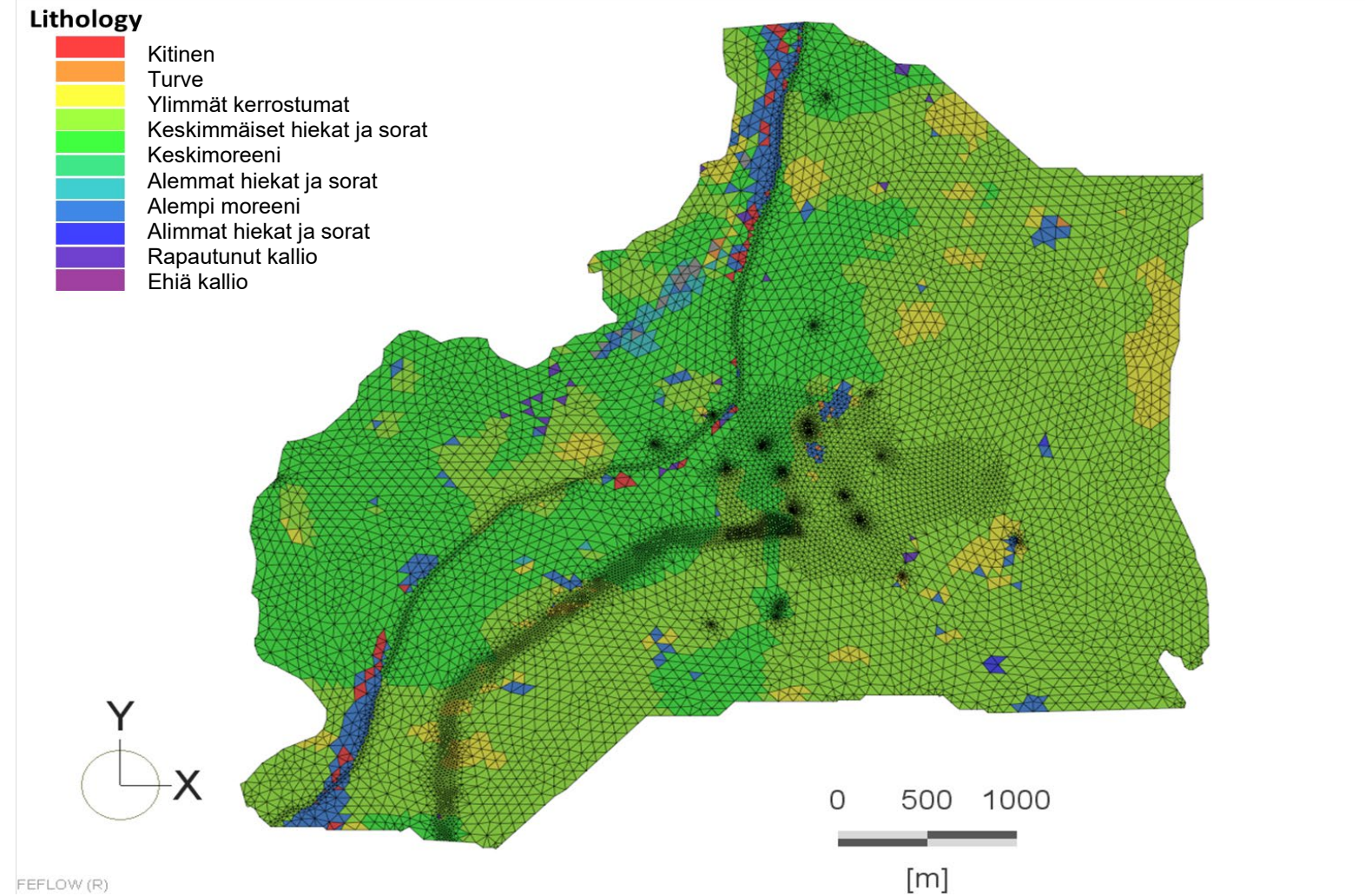
Kuva 6-13 FEFLOW-mallin kerros 4, jossa keskimmäiset hiekat ja sorat (vihreä) länsipuolella ja hajanaisena ylempi moreeni (vaaleanvihreä) itäpuolella
